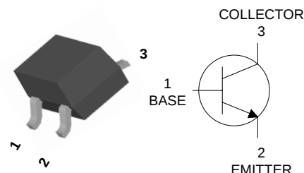
SOT-23
