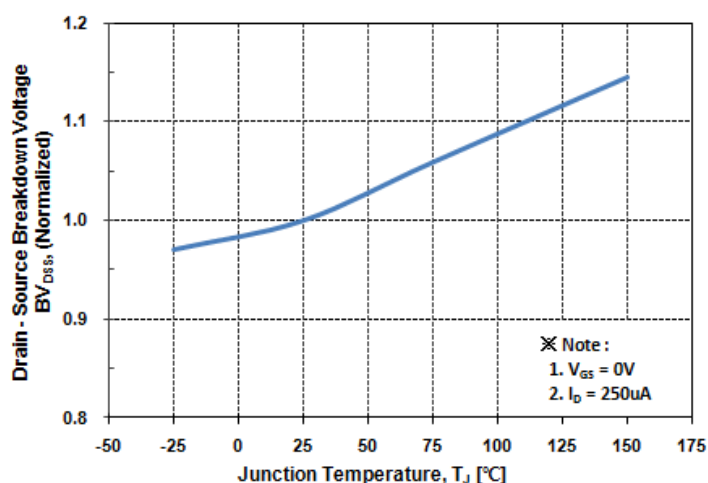
Fig. 7 V_{DS} - T_J
