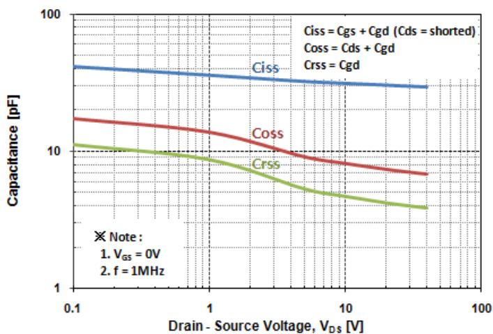
Fig. 5 Capacitance - V_{DS}
