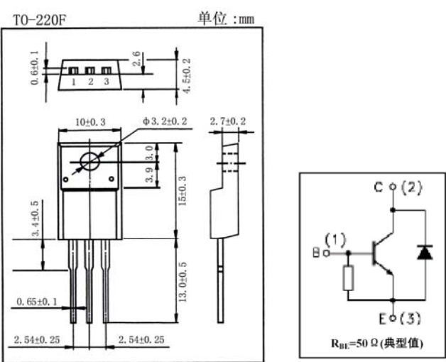
引脚： 1. B 2. C 3. E
