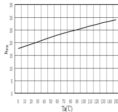
h_{FE}-T_a
