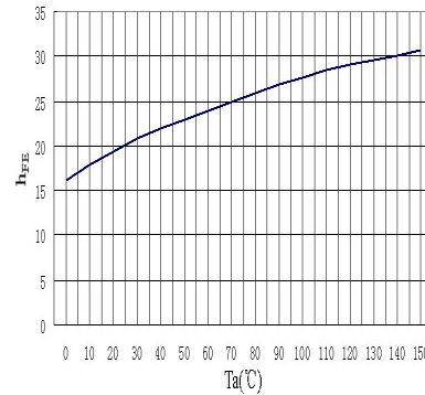
h_{FE}-T_a
