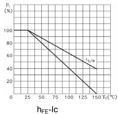
P_C-T_C
