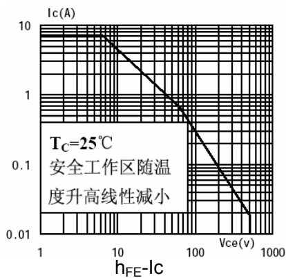
SOA(DC)
