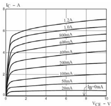
V_{ces}-I_C
