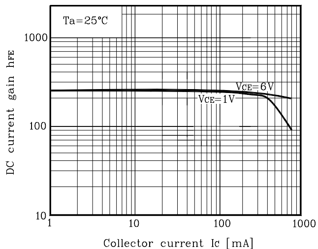
Fig. 5 h_{FE} - I_c
