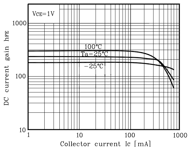
Fig. 6 h_{FE} - I_c
