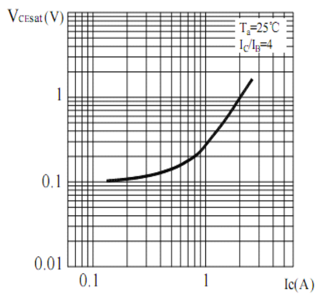
V_{CEsat} \cdot I_C 关系曲线 (典型)
