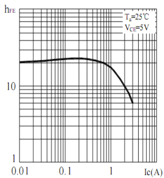
h_{FE} \cdot I_C 关系曲线 (典型)
