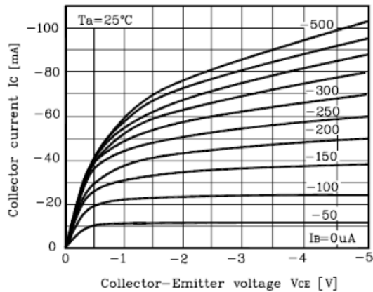
Fig. 3 I_C-V_{CE}
