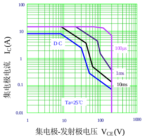
安全工作区（单脉冲）
