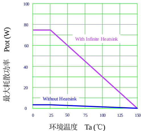
P_{tot} - T_a 关系曲线
