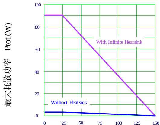
环境温度 T_a (°C)
