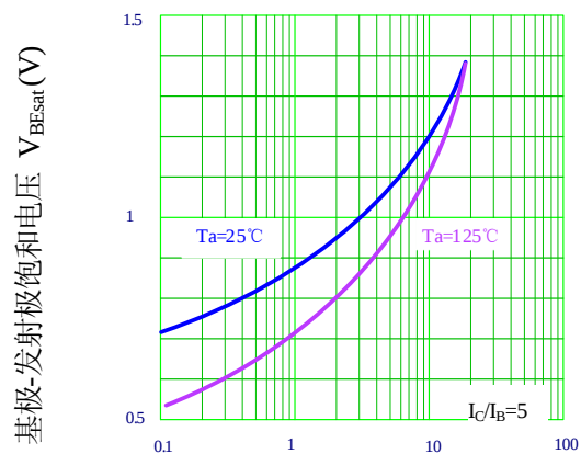
V_{BEsat} - I_C 温度特性 (典型)
