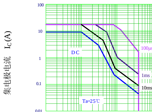
安全工作区（单脉冲）
