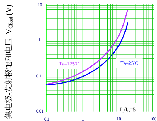
V_{CEsat} - I_C 温度特性 (典型)
