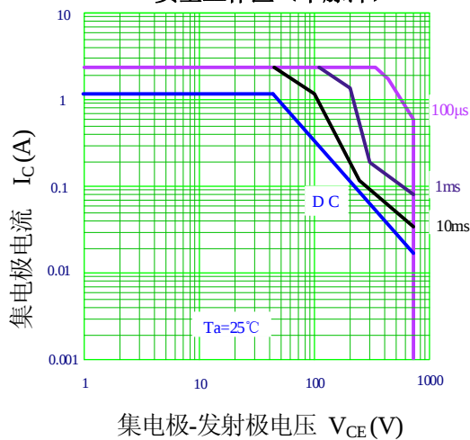
安全工作区 (单脉冲)
