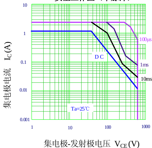
安全工作区 (单脉冲)
