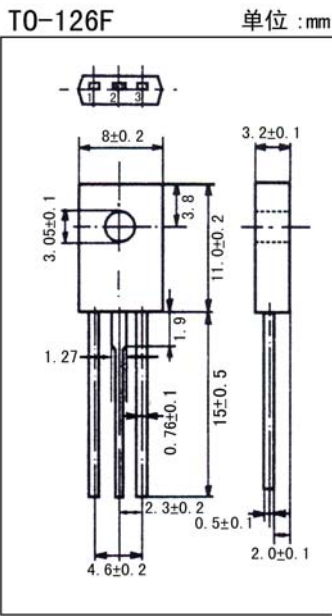
引脚: 1.E 2.C 3.B
