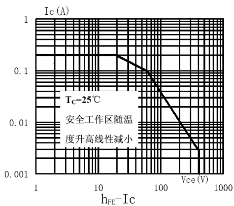
SOA (DC)
