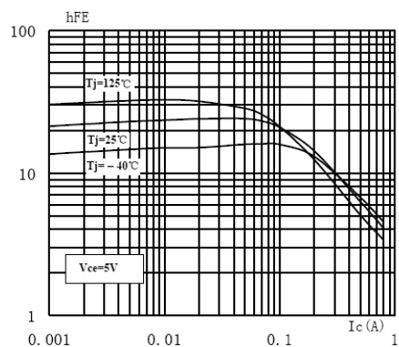
h_{FE}-I_c
