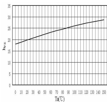
h_{FE}-T_a
