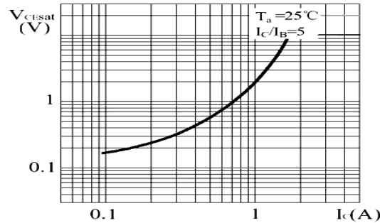
V_{ces} - I_c
