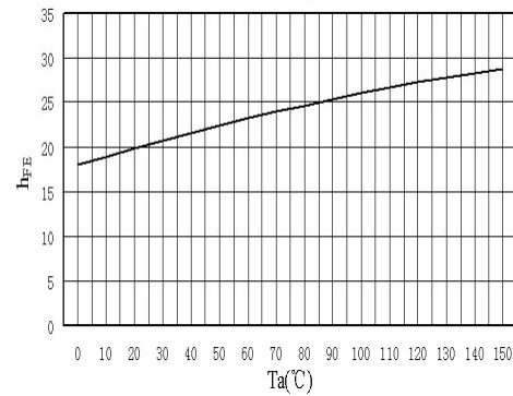
h_{FE} - T_a
