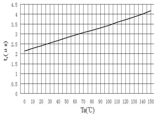
t_s - T_a
