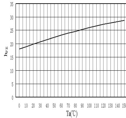
h_{FE}-T_a
