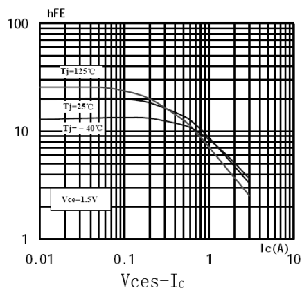
h_{FE} - I_c
