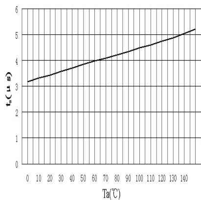
t_s - T_a
