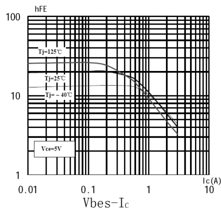
h_{FE} - I_c
