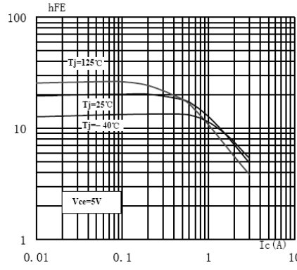
hFE-Ic
