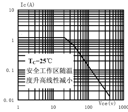
SOA (DC)
