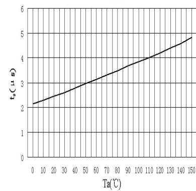
t_s - T_a
