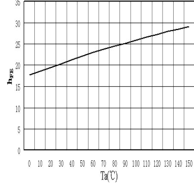
h_{FE} - T_a
