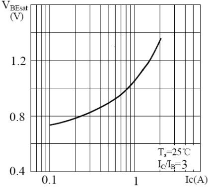
V_{bes}-I_c
