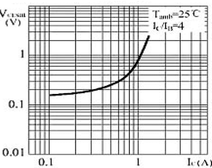
V_{ces} - I_c
