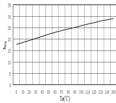
h_{FE}-T_a
