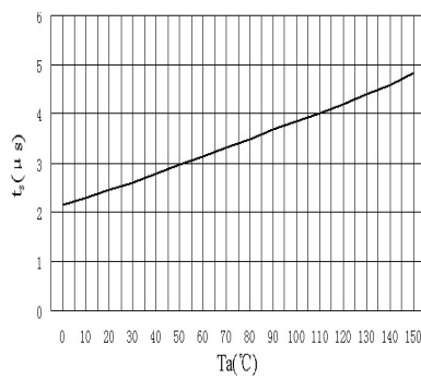
t_s-T_a
