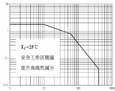
SOA (DC)
