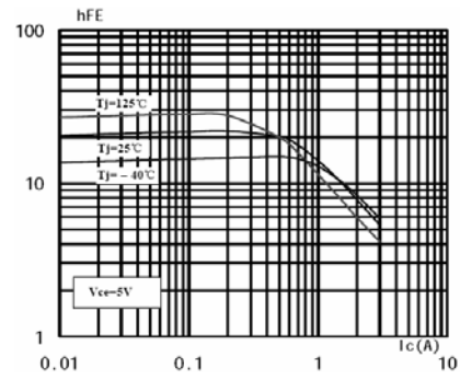
h_{FE}-I_c
