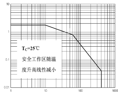
SOA (DC)
