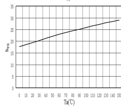
h_{FE}-T_a
