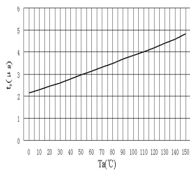
t_s-T_a
