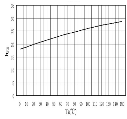
hFE-Ta
