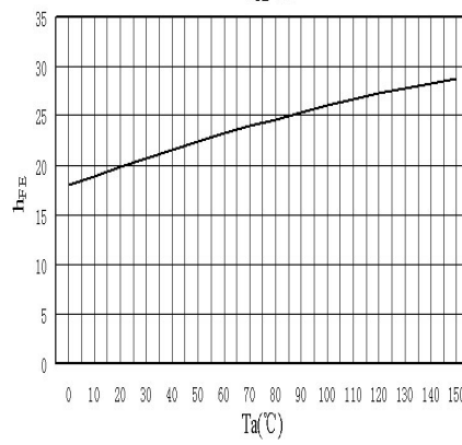
h_{FE}-T_a
