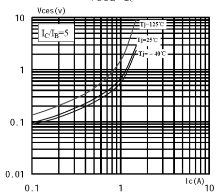
V_{ces}-I_c
