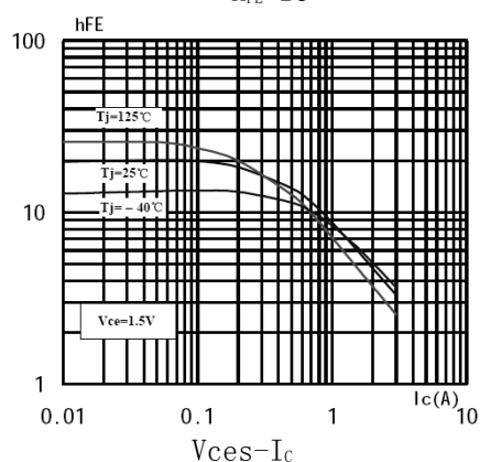
h_{FE}-I_c
