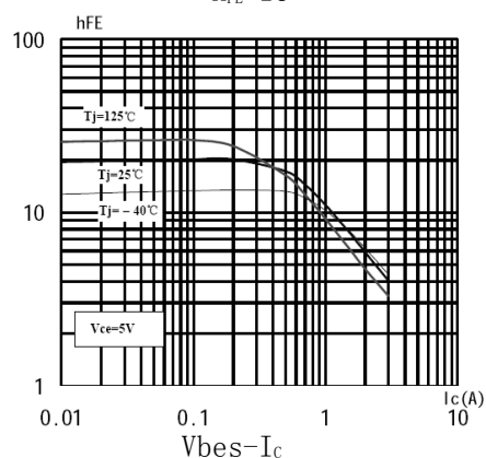
h_{FE}-I_c
