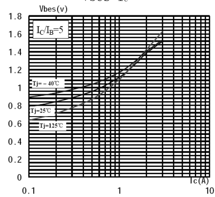
V_{bes}-I_c
