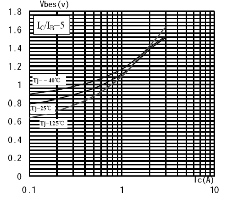
V_{bes}-I_c
