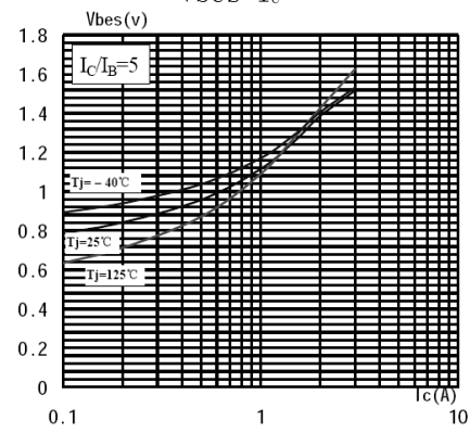
V_{bes} - I_c
