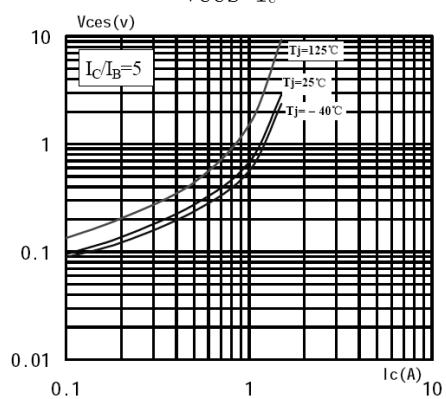
V_{ces} - I_c
