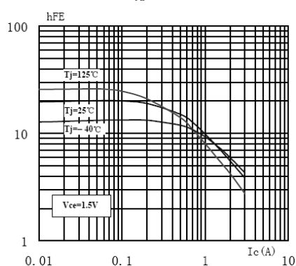
h_{FE} - I_c
