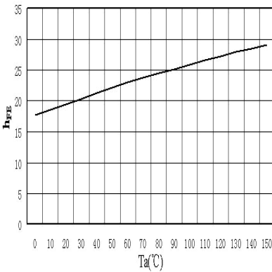
h_{FE} - T_a
