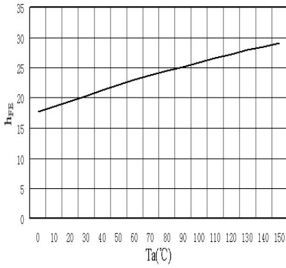
h_{FE}-T_a
