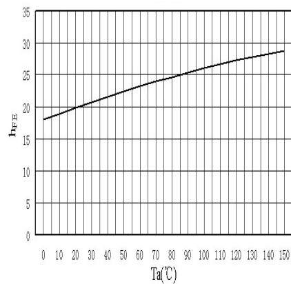
h_{FE}-T_a
