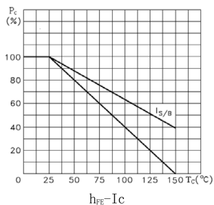
P_C-T_C
