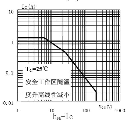
SOA (DC)
