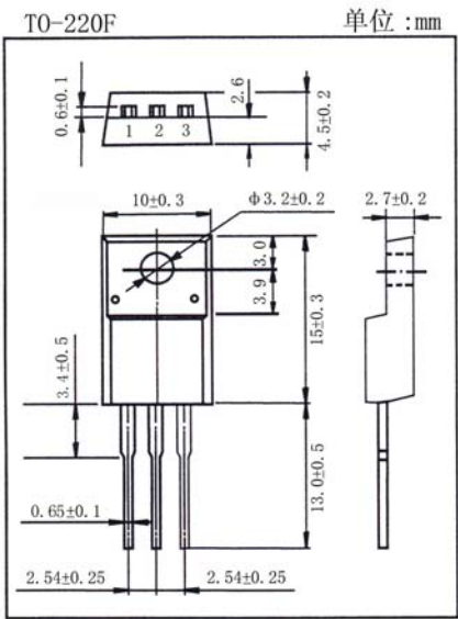
引脚： 1. B 2. C 3. E
