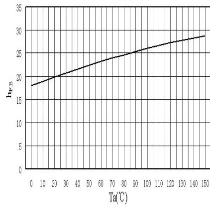
h_{FE}-T_a
