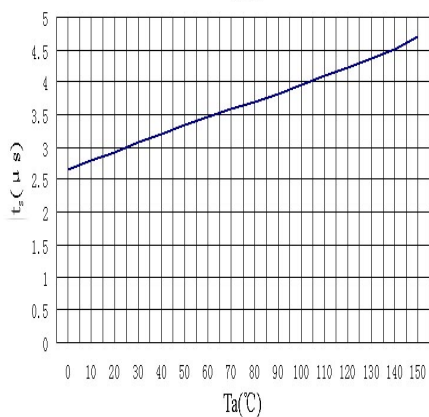
t_s-T_a
