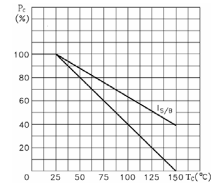
P_c-T_c
