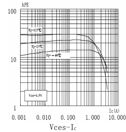
h_{FE}-I_c
