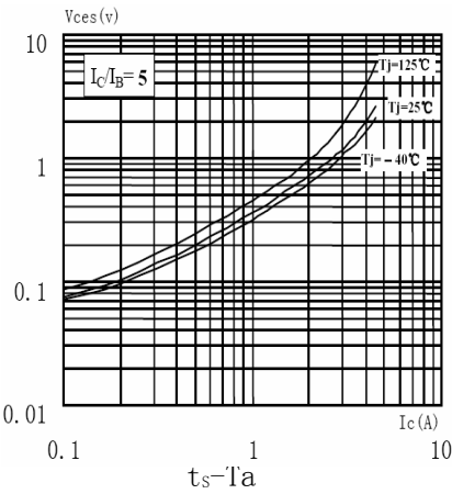
V_{ces}-I_c
