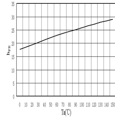
h_{FE}-T_a
