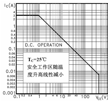
SOA (DC)
