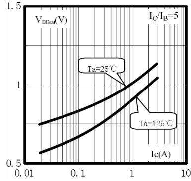
V_{bes}-I_c
