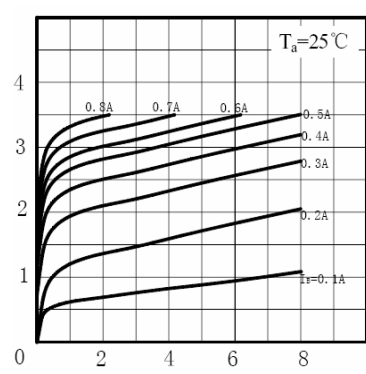
I_c-V_{CE}
