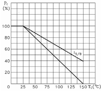
P_c-T_c
