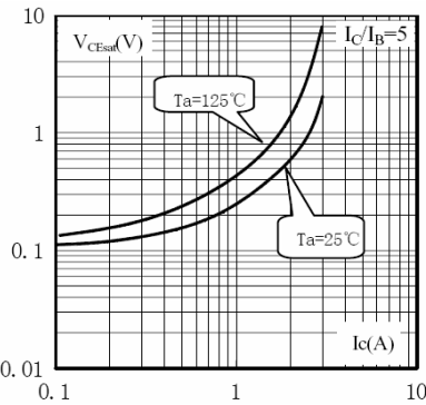
V_{CES}-I_c
