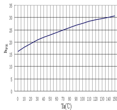
h_{FE}-T_a
