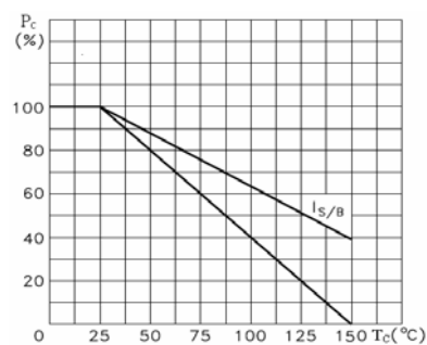
P_c-T_c
