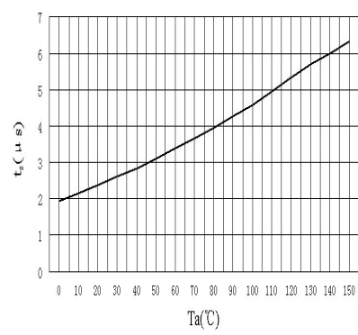
t_s-T_a
