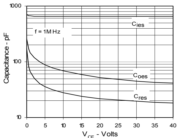
Fig. 12. Capacitance
