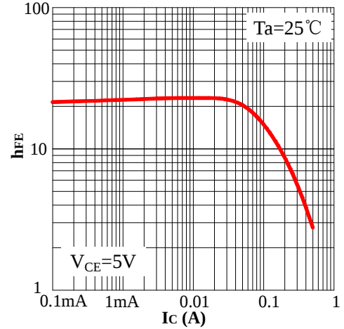
Fig2 h_{FE}-I_C
