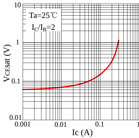
Fig3 V_{CESat}-I_C
