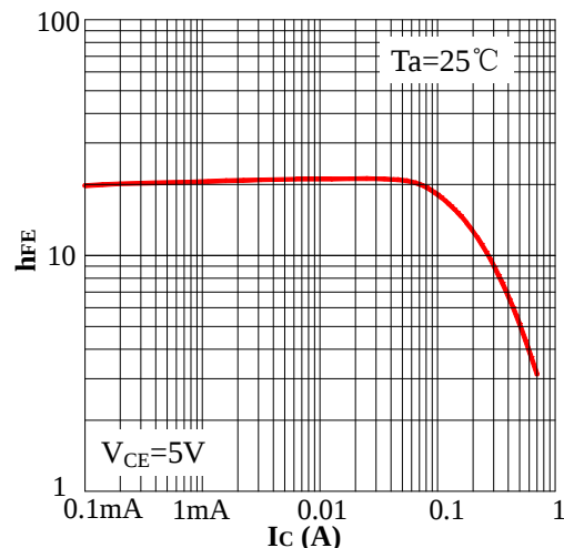
Fig2 h_{FE} - I_C
