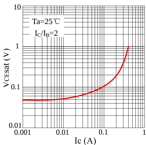
Fig3 V_{CEsat} - I_C
