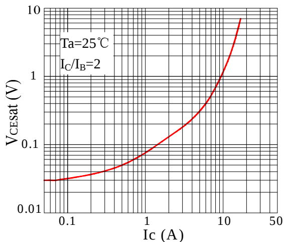
Fig5 VCESat-IC
