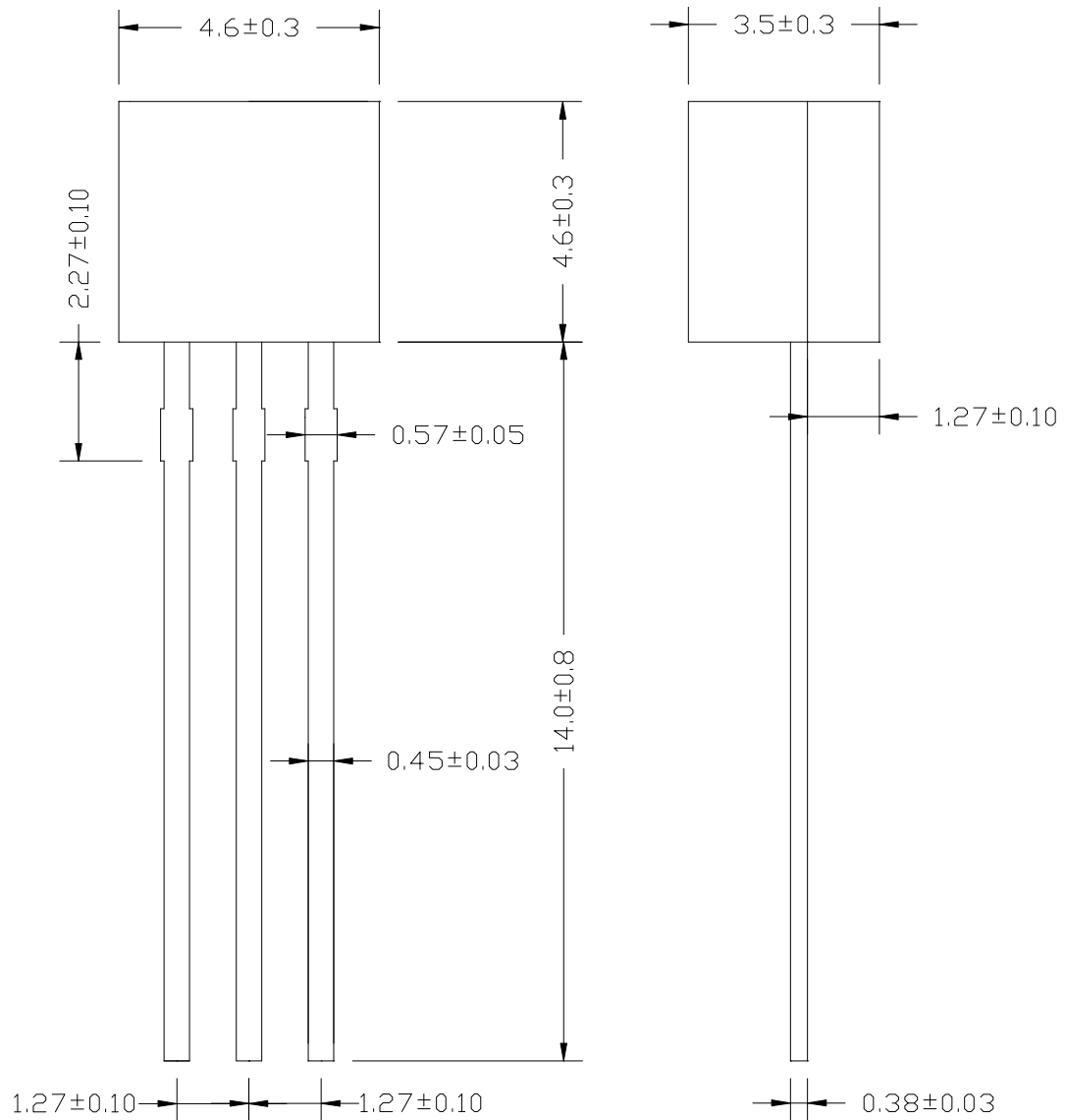
T0-92
