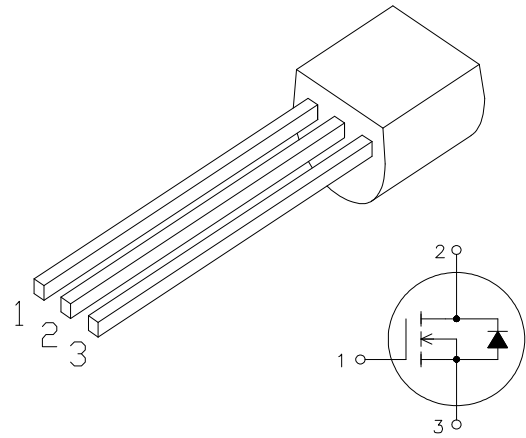
1 栅极(G) 2 漏极 (D) 3 源极(S)
