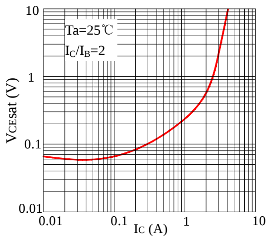
Fig5 VCEsat-IC
