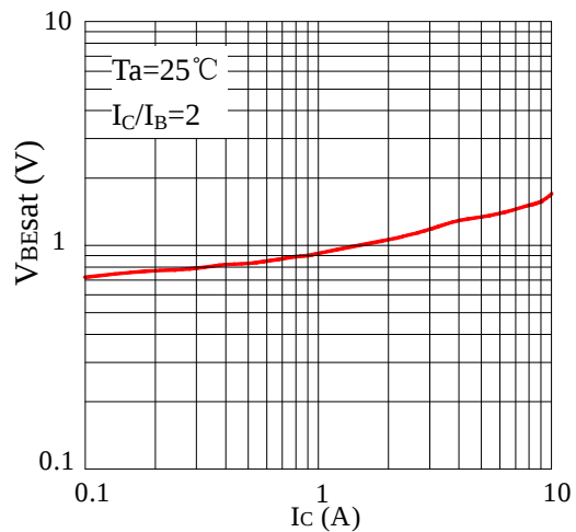
Fig6 VBEsat-IC
