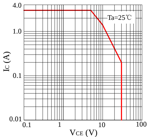
Fig1 SOA (DC)
