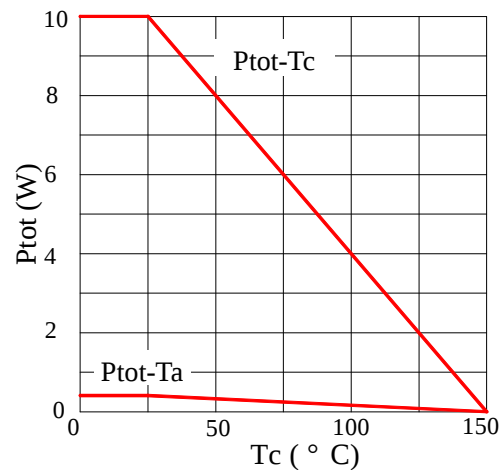
Fig2 Ptot - T
