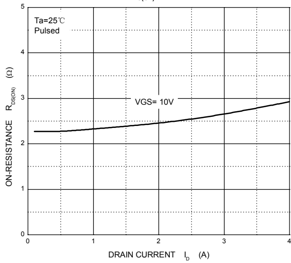
R_{DS(ON)} — I_D
