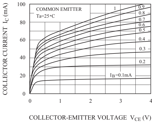
I_C - V_{CE}
