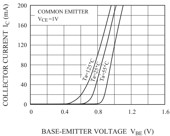
I_C - V_{BE}
