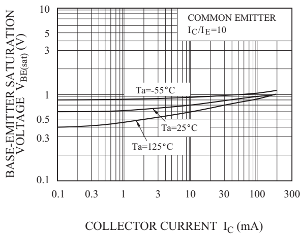
V_{BE(sat)} - I_C
