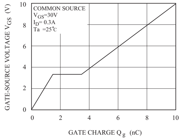
V_{GS} - Q_g
