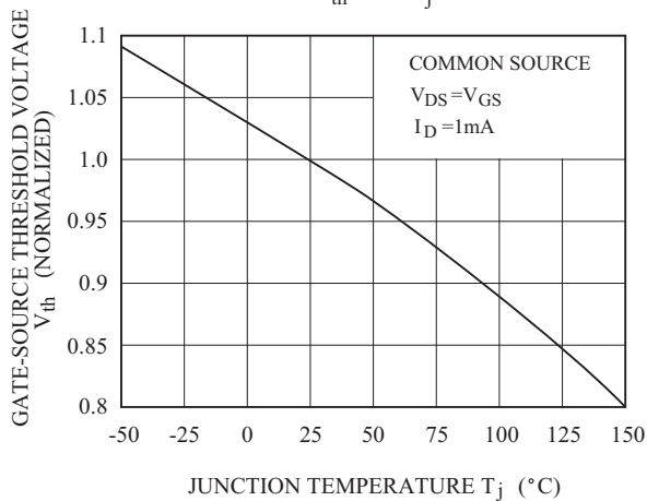
V_{th} - T_j
